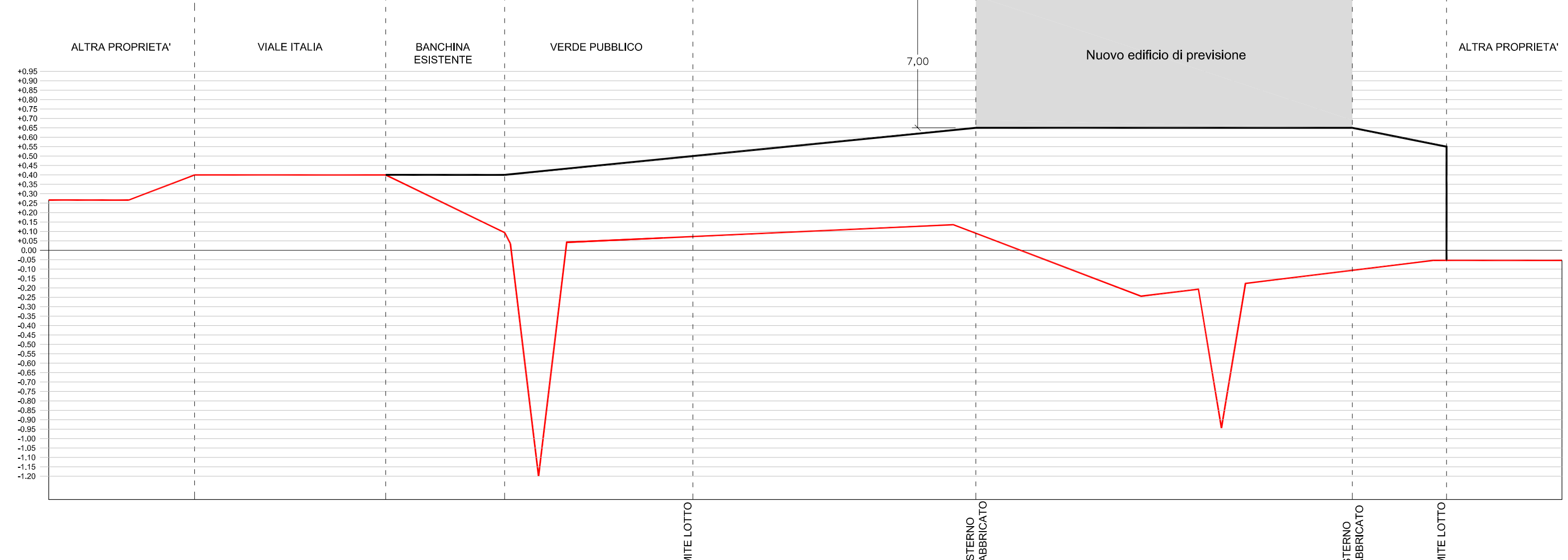
PROFILO 2 SCALA DISTANZE 1:200 SCALA ALTEZZE 1:20 Quota di progetto Quota di campagna
