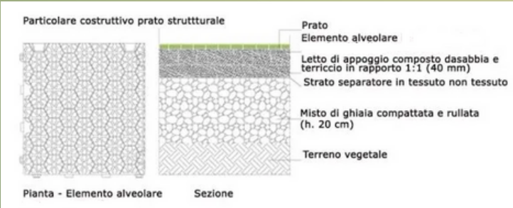
SCHEMA TIPOLOGICO PAVIMENTAZIONE DRENANTE
