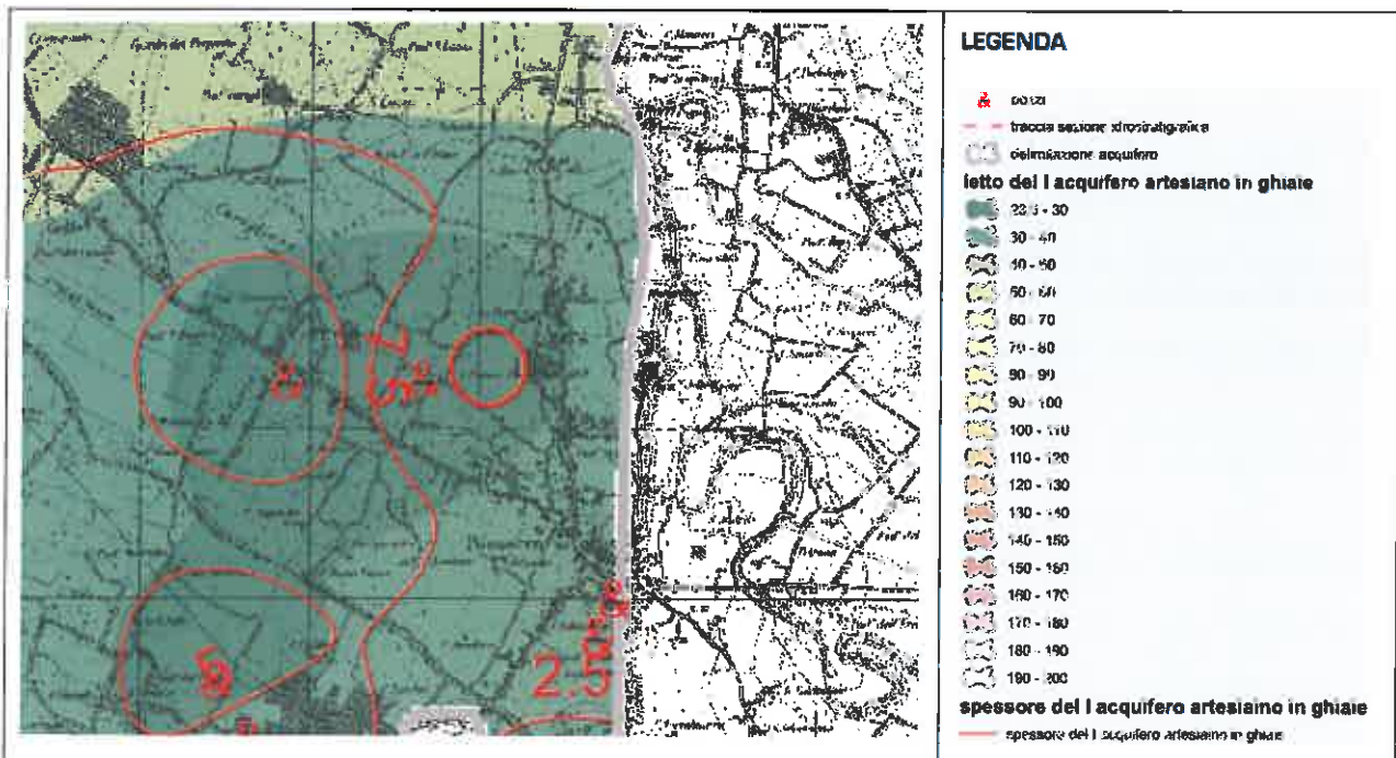
Estratto fuori scala della "Carta del letto e dello spessore del I acquifero artesiano in ghiaie" allegata al Piano di Bacino del Fiume Arno_Stralcio: "Bilancio Idrico" per l'area in esame evidenziata nel cerchio rosso.
