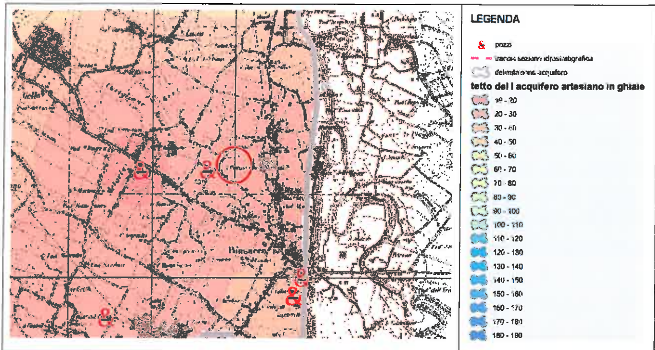
Estratto fuori scala della "Carta della profondità del tetto del I acquifero artesiano in ghiaie" allegata al Piano di Bacino del Fiume Arno_Stralcio: "Bilancio Idrico" per l'area in esame evidenziata nel cerchio rosso.
